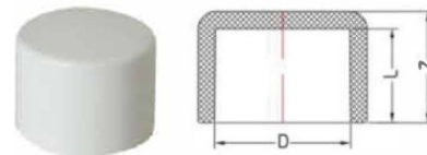
Cap SOC
